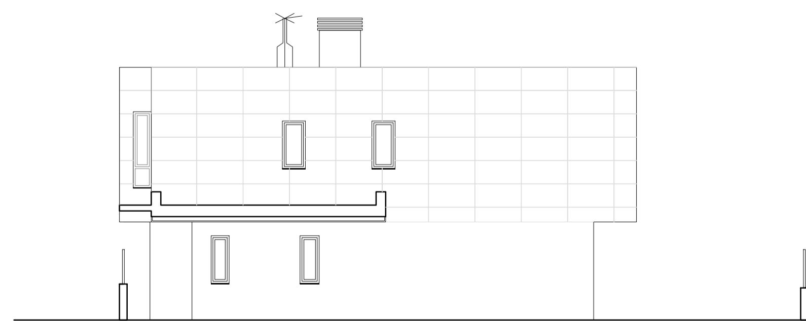
ALZADOS LATERAL TIPO
